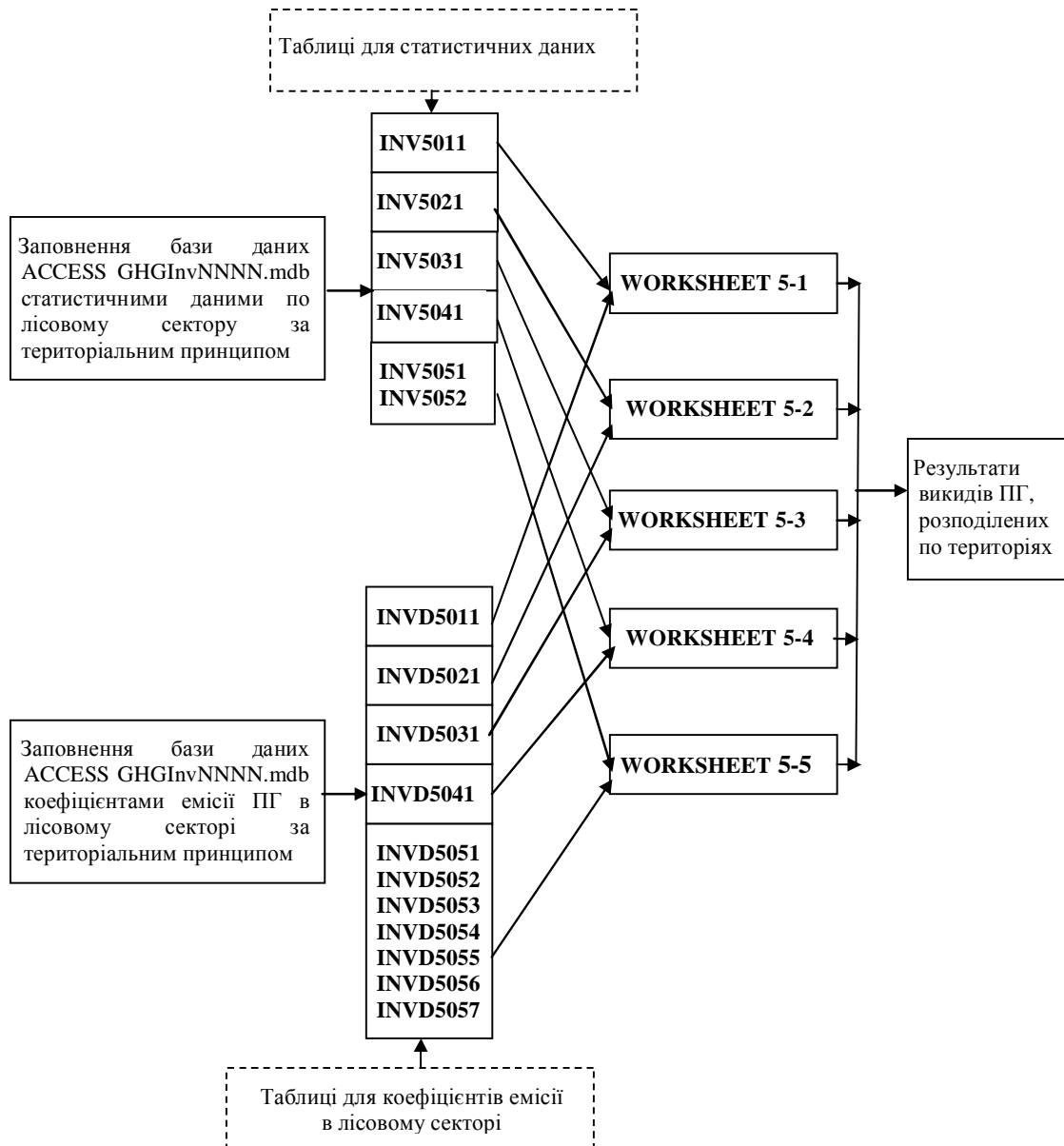
Рис. 5. Структурна схема програмного модуля для обчислення розподіленої інвентаризації в секторі "Лісове господарство"
