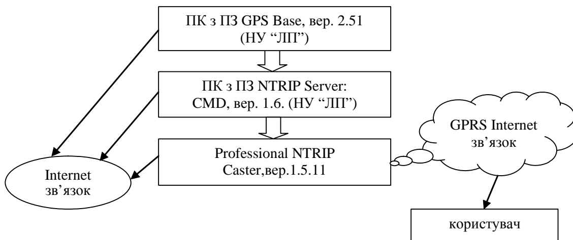
Рис. 2. Схема передавання даних RTK спостережень від постійної станції SULP
