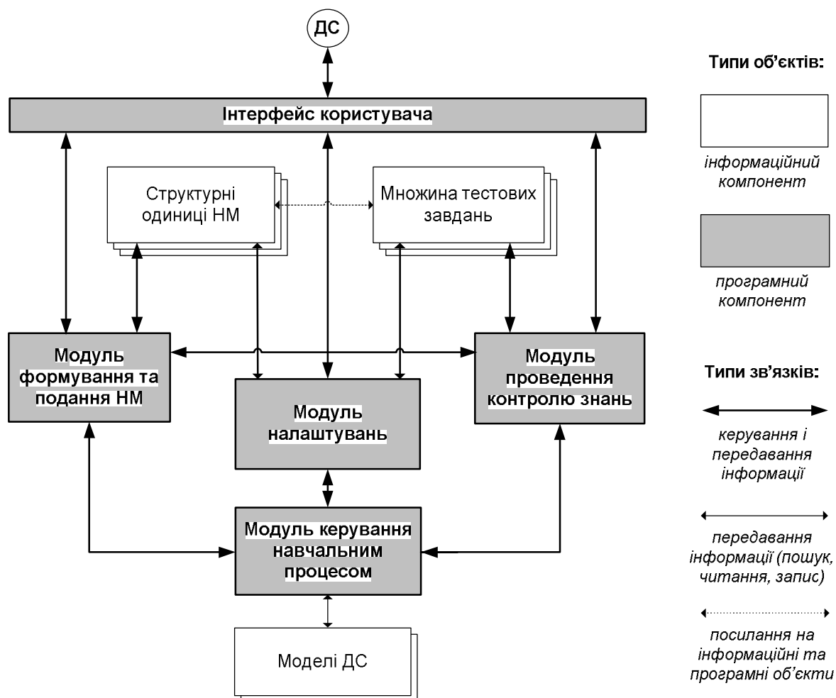
Рис. 6. Схема універсальної архітектури СДМН
