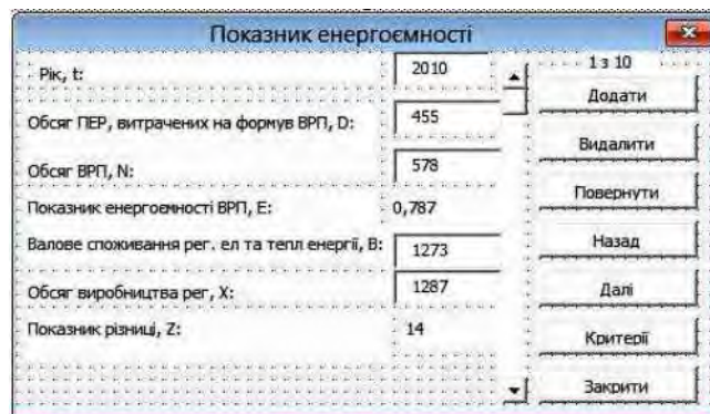
Рис. 2. Форма користувацького інтерфейсу програмного засобу для обчислення показників енергоефективності економіки регіону
