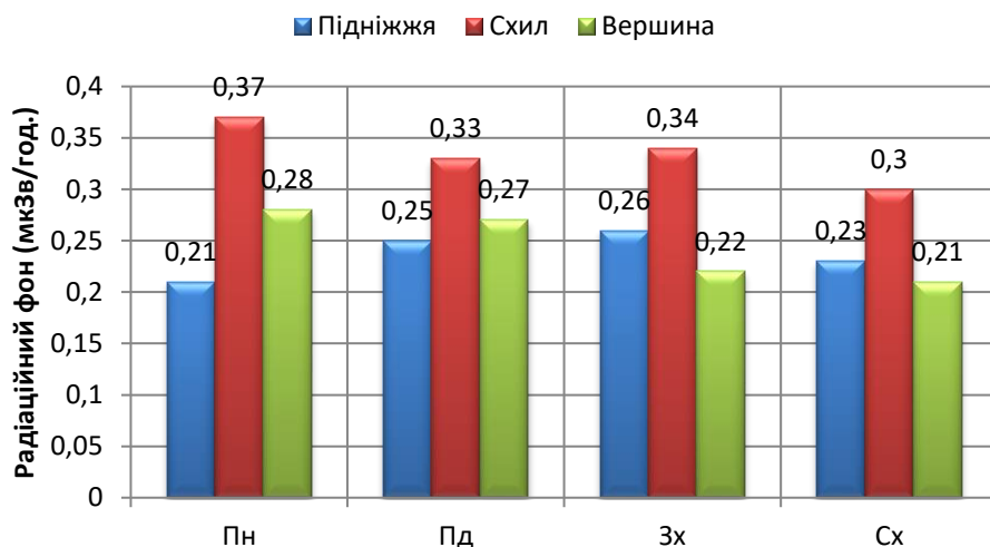
Рисунок 2 – Потужність еквівалентної дози фотонного іонізуючого випромінювання у зоні впливу породного відвалу «Шахти №3 Великомоствівська»
