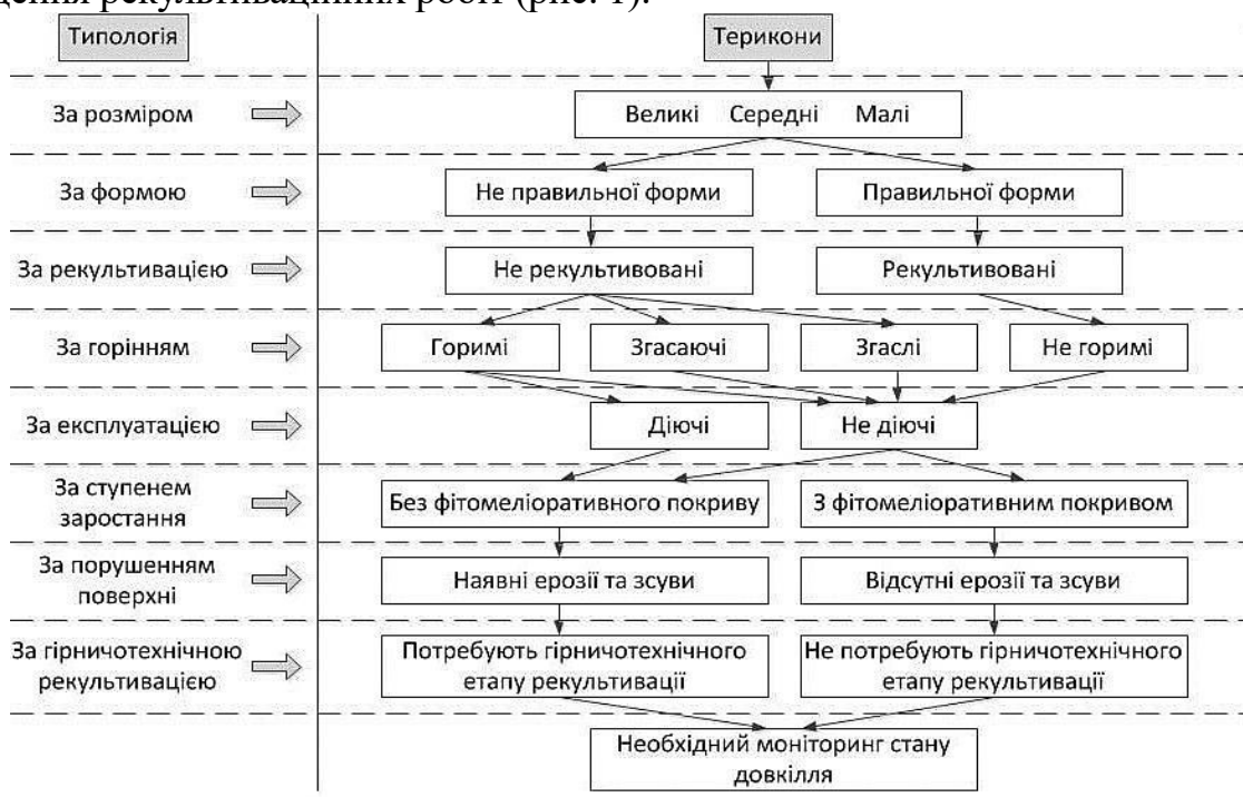
Рисунок 1 – Типологія териконів
