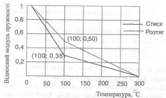
Рис. 1.6. Вплив температури на модуль пружності паралельно до волокон для хвойних порід дерева [8, 12].
