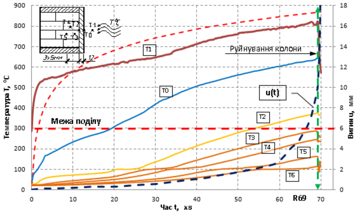
Рис. 3.13. Покази термопар T_i в перерізі дощатоклеєної колони К3.1 і графік деформацій вигину колони u(t) . T_0 \dots T_6 – графіки зміни T(t) на термопарах в часі.
