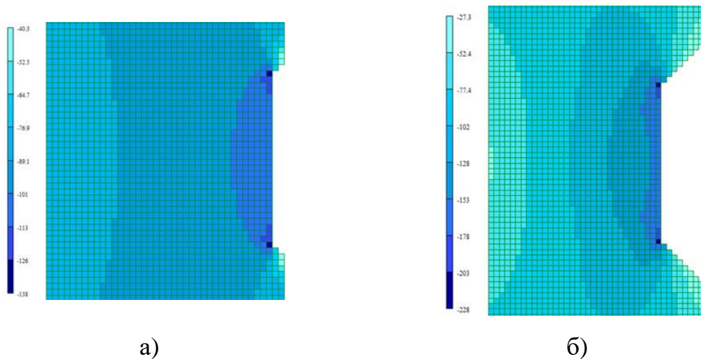
Рис.4.22. Мозаїка напружень в пошкодженому перерізі колони на різних етапах: а) d_{char,n}=5\text{мм} ; б) d_{char,n}=20\text{мм} .
