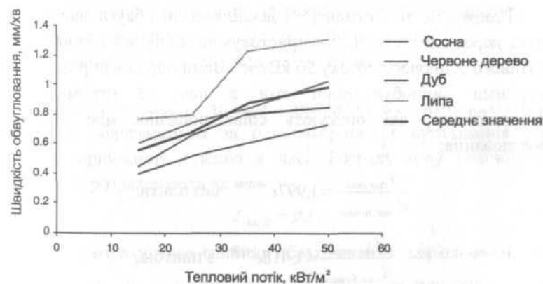
Рис. 1.9. Швидкість обвуглювання деревини [40, 41].
