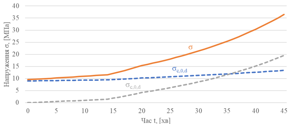
Рис.4.17. Графік залежності напружень \sigma обчислених методом приведеного перерізу від часу t .
