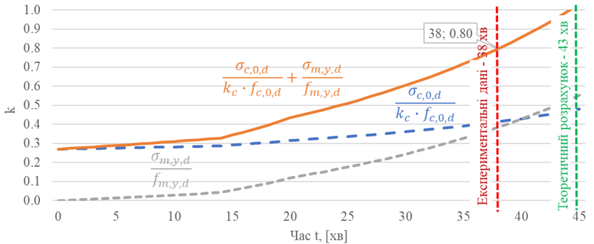
Рис.4.19 Порівняння отриманих теоретичних значень методу приведенного перерізу із експериментальними значеннями для колони К1.1.
