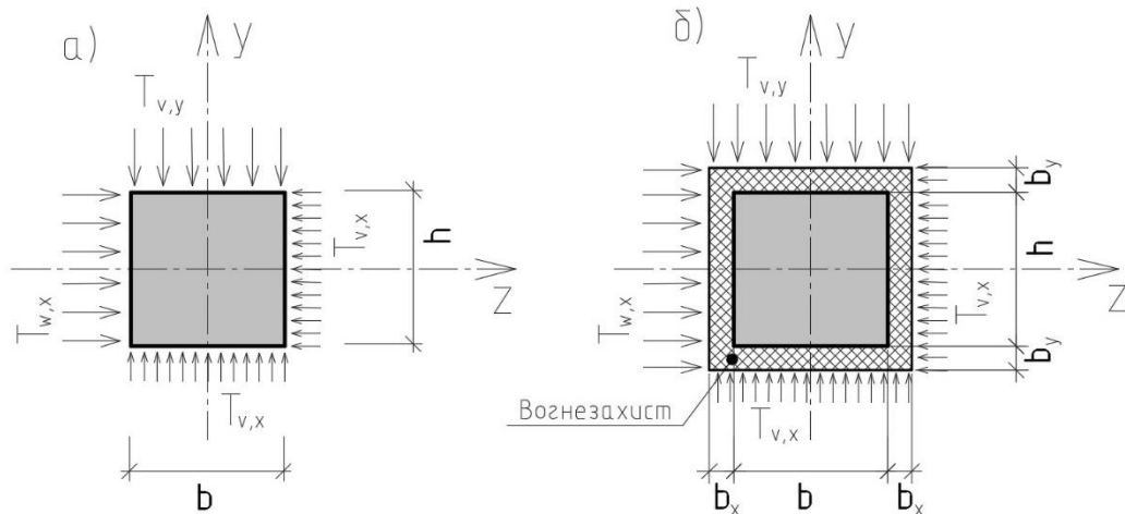
Рис. 4.25. Розрахункова схема температурного поля в колоні.
