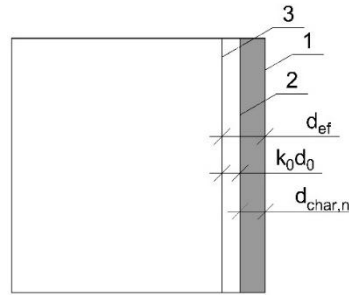
Рис.4.15. Визначення залишкового і робочого поперечного перерізу: 1 – початкова поверхня елемента; 2 – межа залишкового перерізу; 3 – межа робочого поперечного перерізу.
