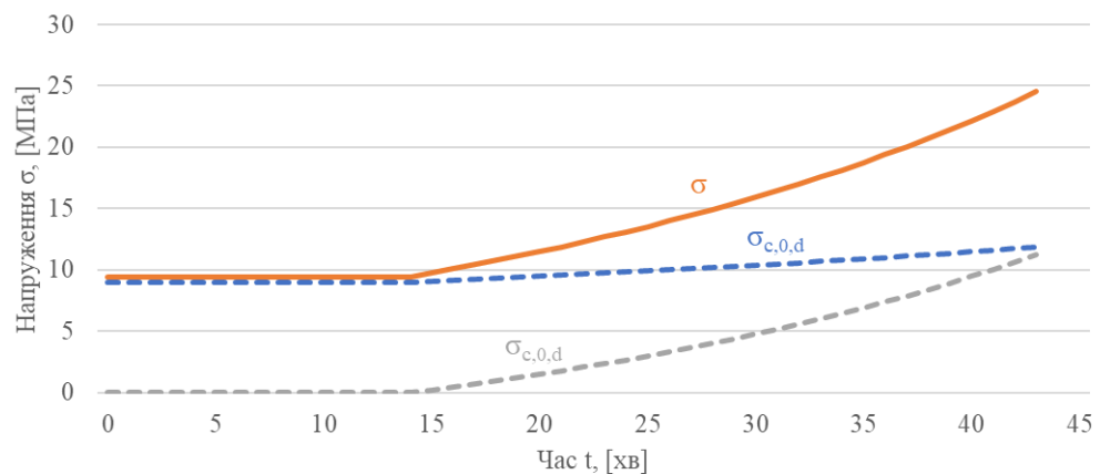
Рис.4.18 Графік залежності напружень \sigma обчислених методом приведених характеристик від часу t .
