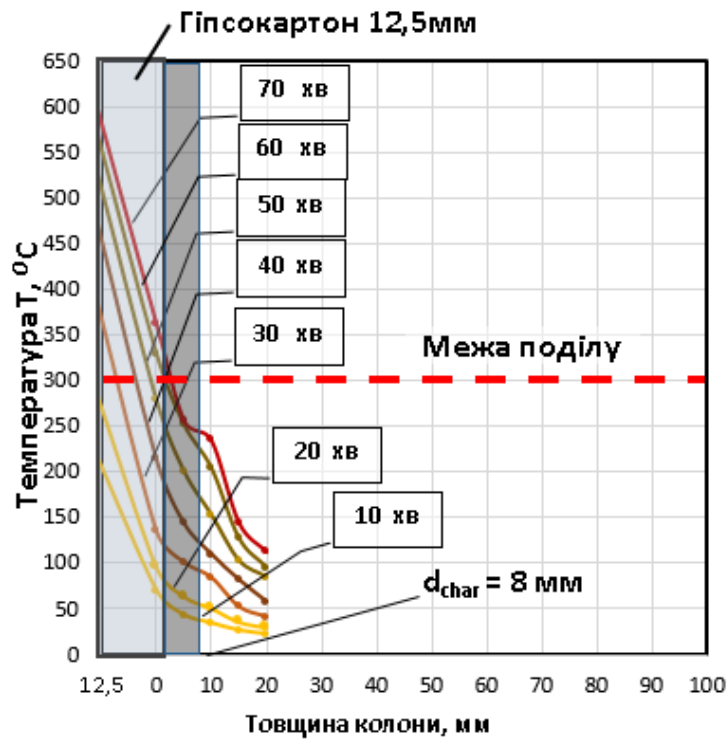
Рис. 3.14. Розподіл температур в перерізі колони К3.1 на різних етапах експерименту
