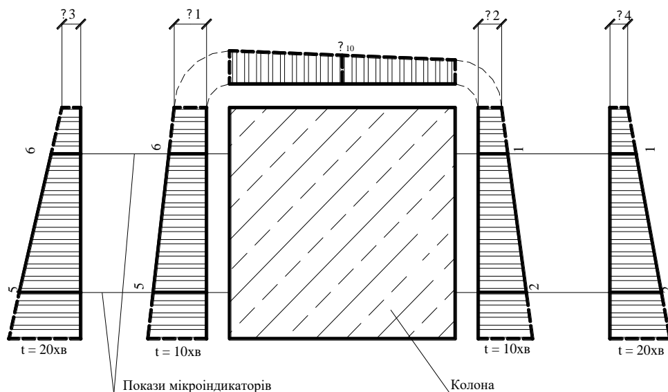
Рис. 3.10 Схема визначення відносних деформацій
