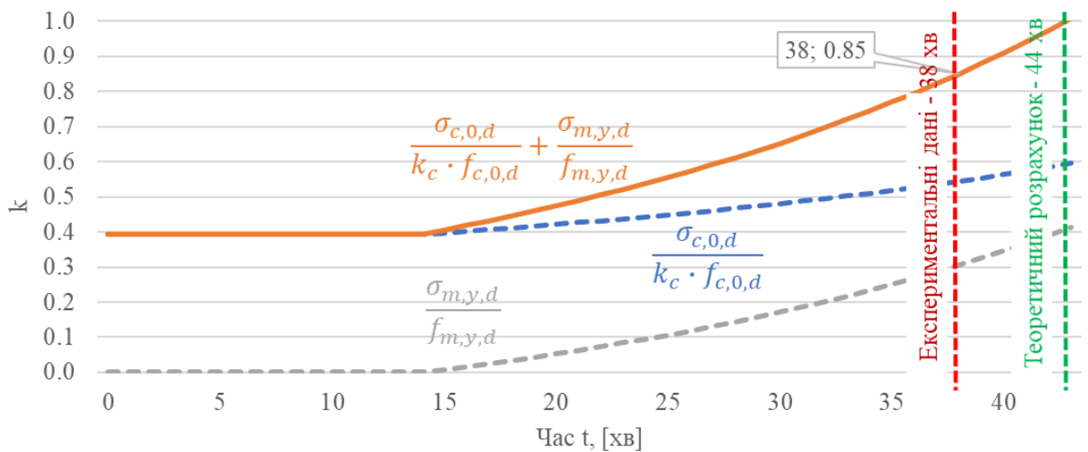
Рис.4.20 Порівняння отриманих теоретичних значень методу приведених характеристик із експериментальними значеннями для колони К1.1.
