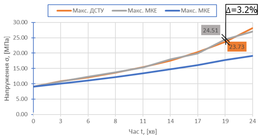
Рис.4.23. Порівняння напружень обчислених методом скінчених елементів та максимальний напружень обчислених методом приведенного перерізу.
