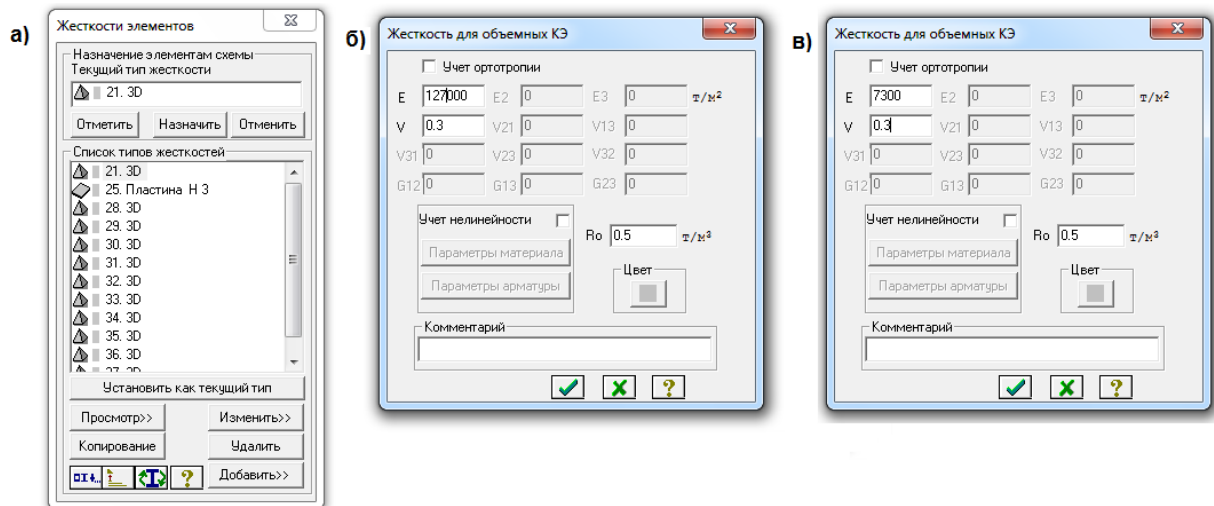
Рис. 4.8. Жорсткості об'ємних кінцевих елементів моделі колони: а) загальний список; б) при температурі 20 °С; в) при температурі 200 °С
