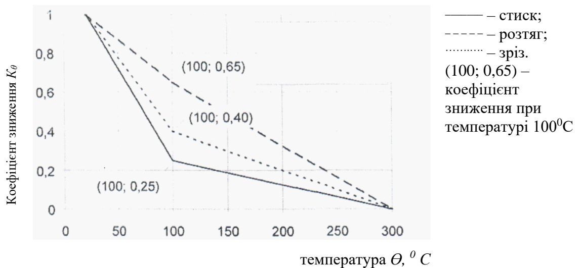
Рис. 4.3. Залежності зміни коефіцієнтів зниження міцності K_\theta деревини на стиск, розтяг і зріз від температури.
