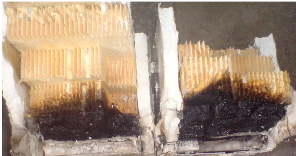
Рис. 3.12. Вигляд дощатоклеєних колон після руйнування на сумісну дію осевого навантаження та локального нагріву
