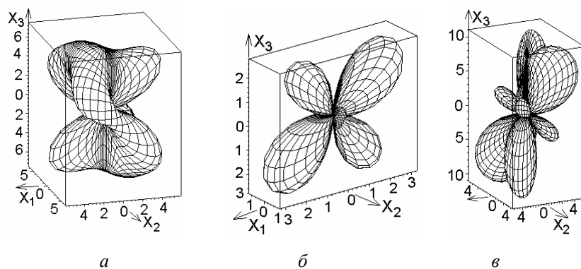
Рис. 4. Вказівні поверхні поздовжнього \pi'_{ii} (а) і поперечного \pi'^{(i)}_{im} (б), \pi'^{(m)}_{im} (в) ПОЕ у моноклінних кристалах тригліцинсульфату ТГС (клас симетрії 2 ); усе – Бр
