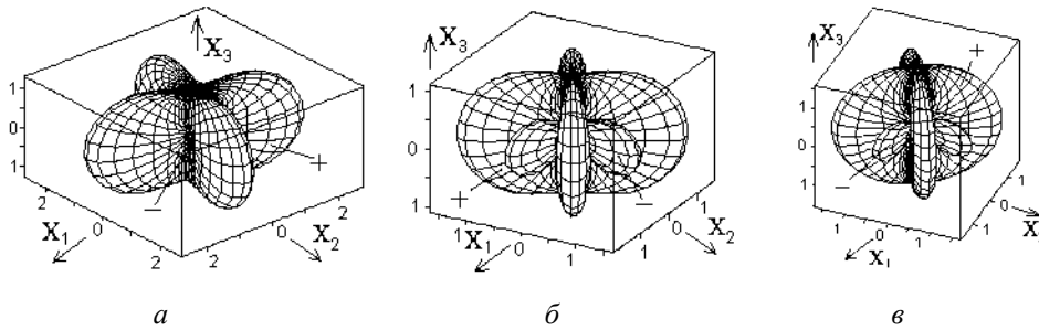
Рис. 3. Вказівні поверхні поздовжнього \pi'_{ii} (а) і поперечного \pi'^{(i)}_{im} (б), \pi'^{(m)}_{im} (в) ПОЕ у тетрагональних кристалах вольфрамату кальцію \text{CaWO}_4 (клас симетрії 4/m ); усе – Бр
