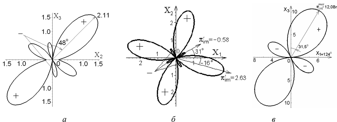
Рис. 5. Перерізи головними площинами ВП поздовжнього ПОЕ \pi'_{ii} кристалів ніобату літію (а), вольфраму кальцію (б) та переріз площиною X_3, X_{1+124}^\circ поперечного ПОЕ \pi'_{im}^{(m)} кристалів ТГС (в); усе – Бр
