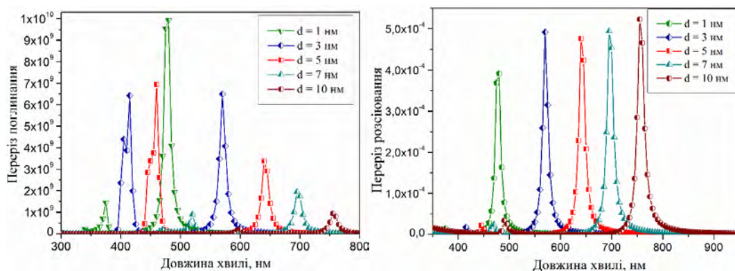
Рис. 9. Вплив товщини оболонки (діоксид титану) наноеліпсоїда (срібло) на спектральне положення й амплітуду плазмонного резонансу, що міститься у середовищі із показником заломлення 1,33, осі еліпсоїда a=15 нм, b=10 нм
