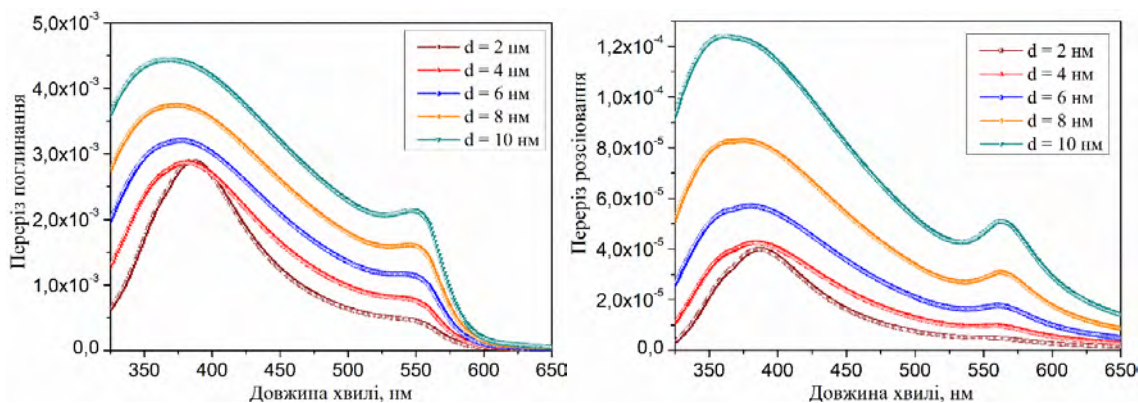
Рис. 4. Вплив товщини мідної оболонки на спектральні характеристики сферичної наночастинки Ag діаметром 30 нм, розташованої у середовищі із показником заломлення 1,33
