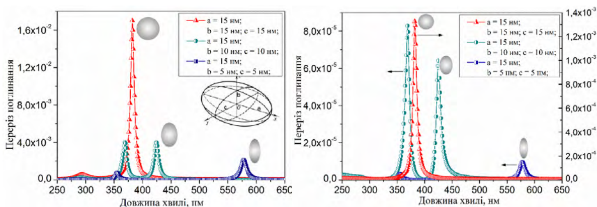
Рис. 6. Вплив співвідношення розміру осей на спектральні характеристики срібного наноеліпсоїда, що міститься у середовищі із показником заломлення 1,33
