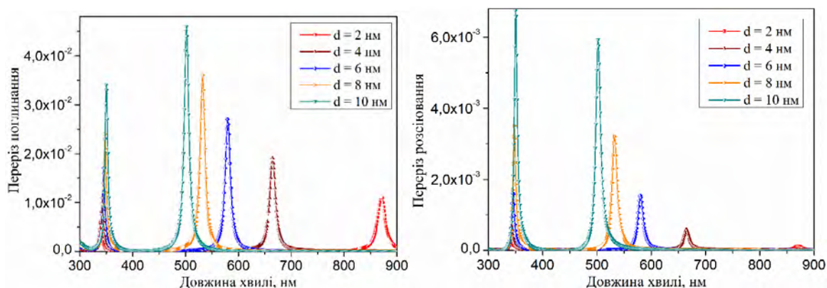
Рис. 5. Вплив товщини срібної оболонки на спектральні характеристики сферичної наночастинки \text{TiO}_2 діаметром 30 нм, що міститься у середовищі із показником заломлення 1,33
