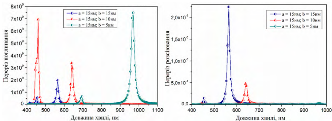
Рис. 7. Вплив співвідношення розміру осей наноеліпсоїда (срібло) із оболонкою (діоксид титану) на спектральне положення й амплітуду плазмонного резонансу, що міститься у середовищі із показником заломлення 1,33, товщина оболонки 5 нм
