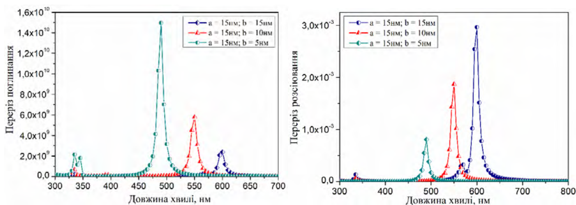
Рис. 8. Вплив співвідношення розміру осей наноеліпсоїда (діоксид титану) з оболонкою (срібло) на спектральне положення й амплітуду плазмонного резонансу, що міститься у середовищі з показником заломлення 1,33, товщина оболонки 5 нм
