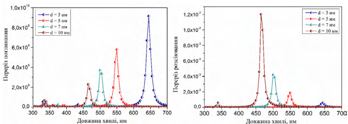
Рис. 10. Вплив товщини оболонки (срібло) наноеліпсоїда (діоксид титану) на спектральне положення і амплітуду плазмонного резонансу, що міститься у середовищі із показником заломлення 1,33, осі еліпсоїда a=15 нм, b=10 нм
