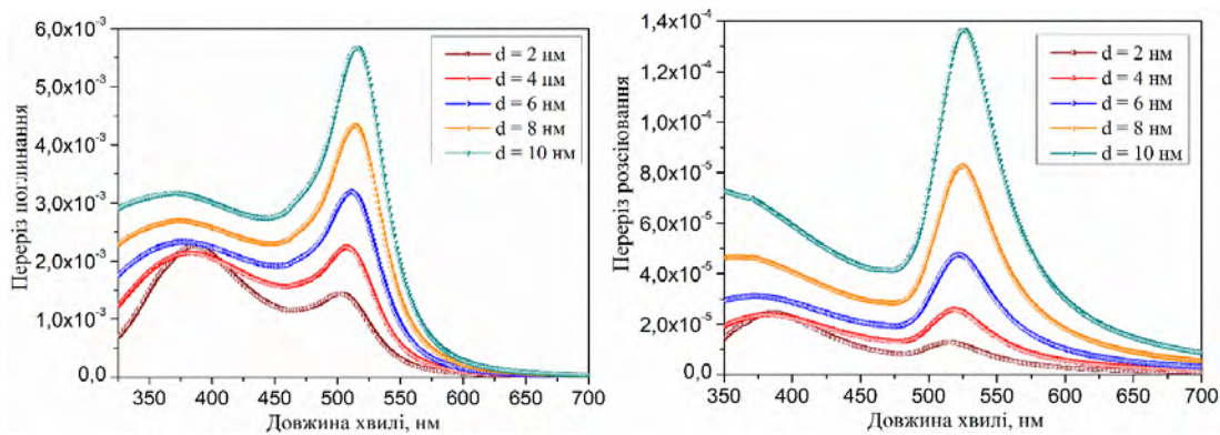
Рис. 3. Вплив товщини золотої оболонки на спектральні характеристики сферичної наночастинки Ag діаметром 30 нм, що міститься у середовищі із показником заломлення 1,33
