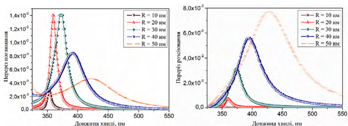
Рис. 1. Вплив радіуса на спектральне положення та амплітуду плазмонного резонансу сферичної наночастинки срібла, що міститься у середовищі із показником заломлення 1,0027
