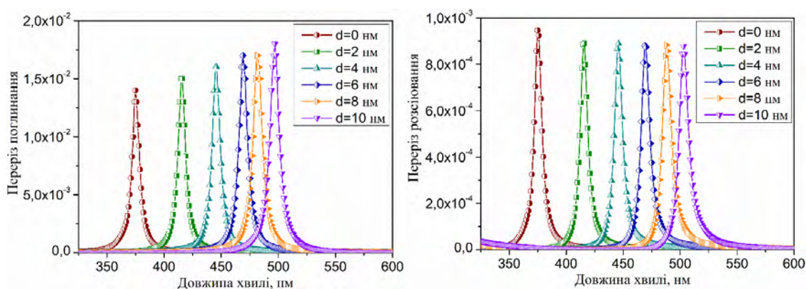
Рис. 2. Вплив товщини оболонки TiO 2 на спектральні характеристики сферичної наночастинки срібла діаметром 30 нм, що міститься у середовищі із показником заломлення 1,33
