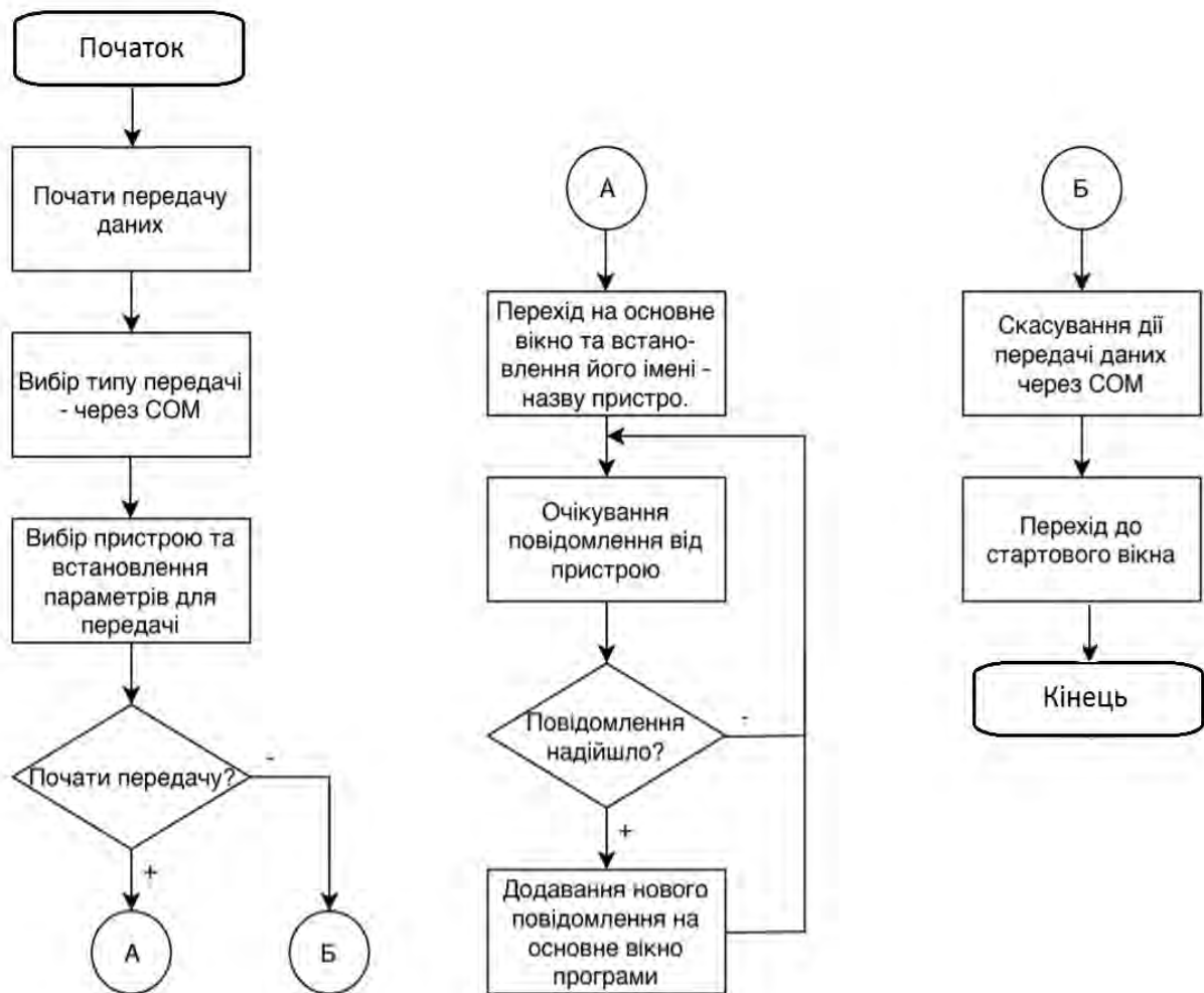
Рис. 3. Алгоритм з'єднання та роботи з COM-пристроєм
