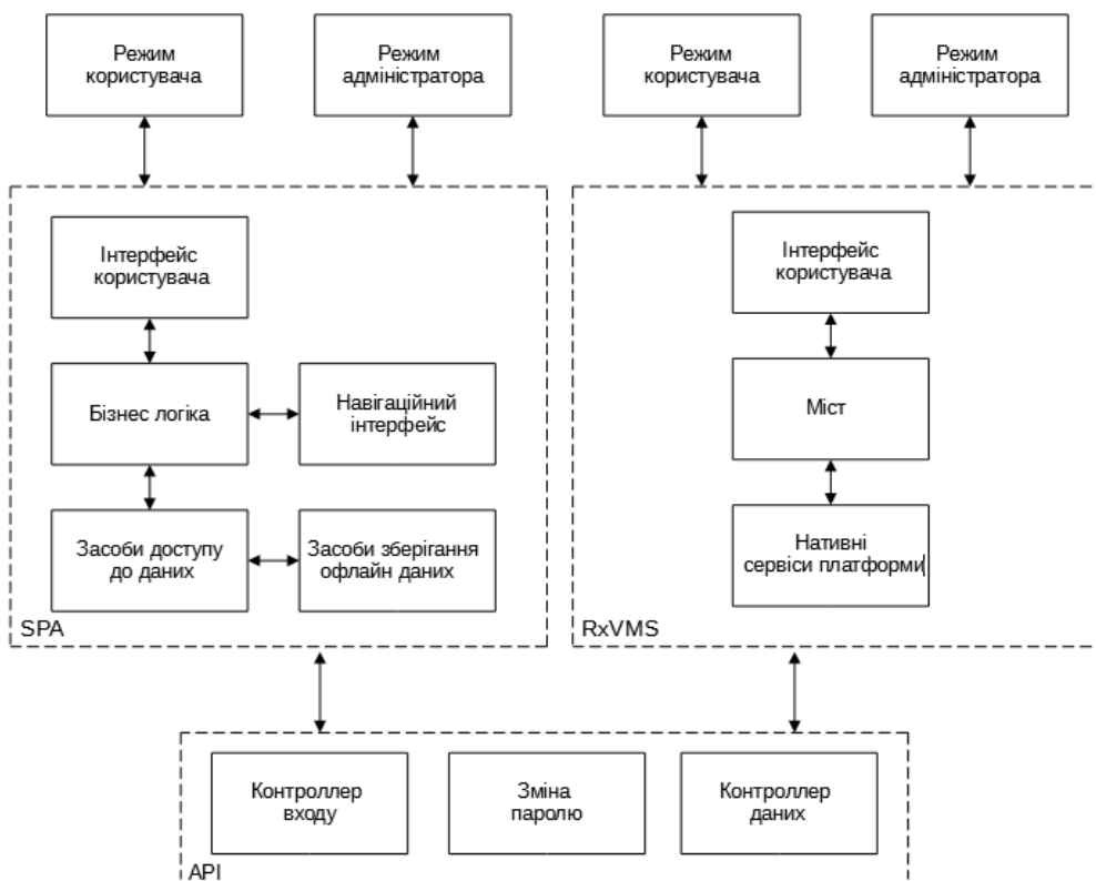
Рис. 5. Структура зв'язків клієнтської частини
