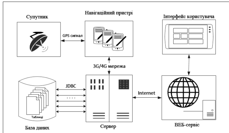
Рис. 1. Загальна структура кіберфізичної системи
