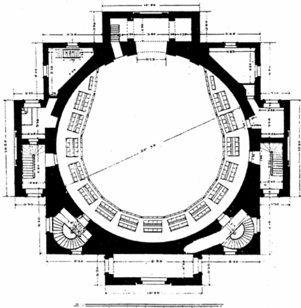
Рис. 8. Синагога Тимпель. Архівне фото, архівні креслення головного фасаду та плану 1-го поверху
