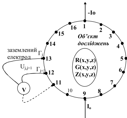
Рис. 4. Полусный метод збудження
