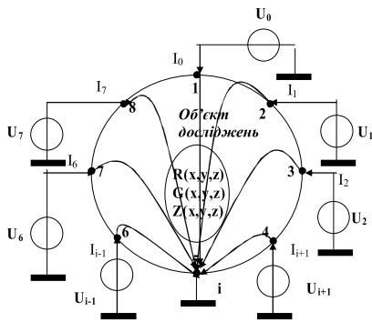
Рис. 1. Оксфордська схема методу вимірювань в електричній томографії
