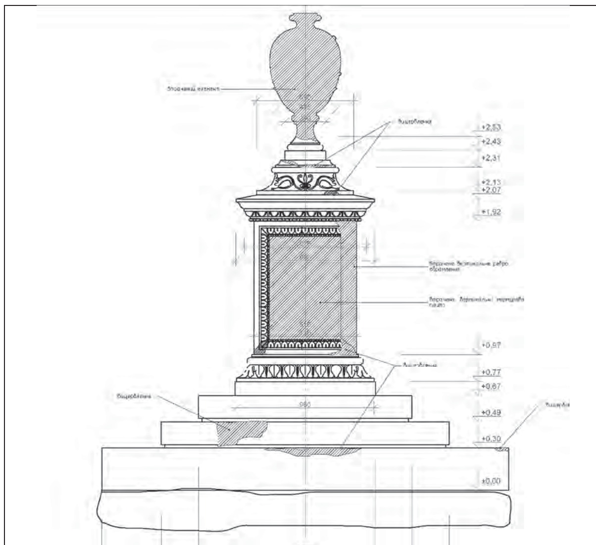
Лл. 8. Проектна документація з еставації надгробного пам'ятника на Личаківському цвинтарі професора Львівської політехніки, ректора Юліана Захарівича. Картограма втрат та технічного стану. Північний фасад пам'ятника. Опрацювання: асп. З. Лукомська, К. Присяжний, кер. М. Бевз, 2006 р.
