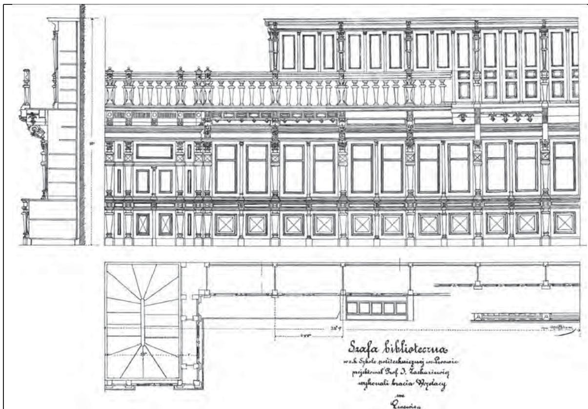
Лл. 2. Архівне креслення авторства Ю. Захаревича шафи для бібліотеки у головному корпусі Політехніки. Нині це приміщення № 214 головного корпусу. Верхній ярус шаф втрачено у радянський період. У 2017 році спеціалісти кафедри виконали дослідження приміщення та науково-проектну документацію з відтворення автентичного інтер'єру та умеблювання і пристосування його на функцію Зали урочистих церемоній Львівської політехніки
