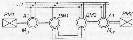
Рис. 1. Функціональна схема.
