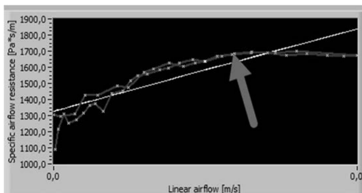
Рис. 3. Зв'язок між лінійним потоком повітря та питомим опором повітряного потоку
