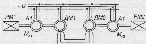
Рис. 1. Функціональна схема
