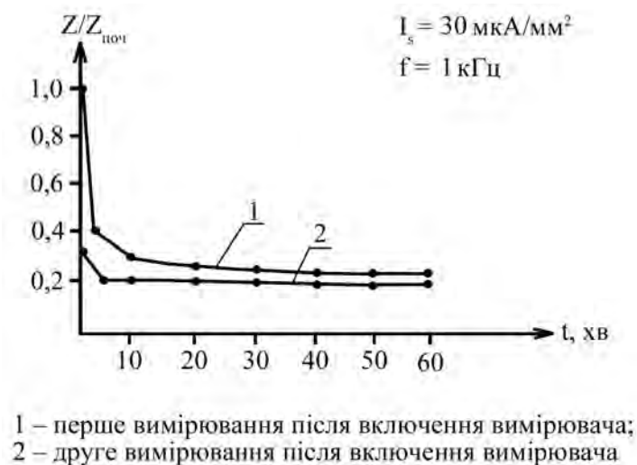
Рис. 4. Характерна зміна ступеня нестабільності міжелектродного імпедансу після початку роботи вимірювача
