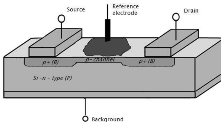
Fig. 1. ISFET structure
