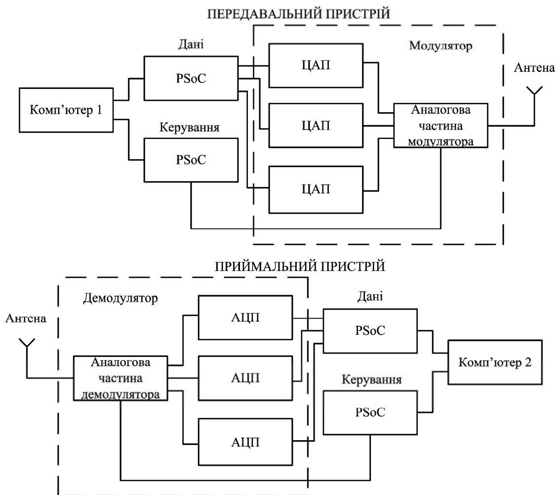
Рис. 4. Структурна схема вискоєфективної системи, основаної на використанні АМБС
