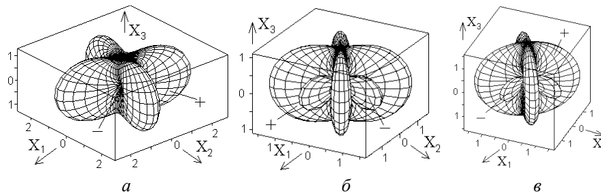
Рис. 3. Вказівні поверхні поздовжнього \pi'_{ii} (а) і поперечного \pi'^{(i)}_{im} (б), \pi'^{(m)}_{im} (в) ПОЕ в тетрагональних кристалах вольфраму кальцію \text{CaWO}_4 (клас симетрії 4/m ); усе в од. Бр
