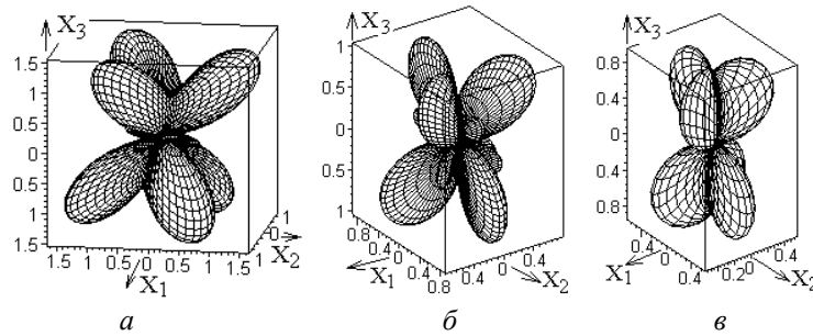
Рис. 2. Вказівні поверхні ПОЕ тригональних кристалів ніобату літію \text{LiNbO}_3 (клас симетрії 3m ): а – поверхня \pi'_{ii} поздовжнього ПОЕ, б – поверхня поляризації світла \pi'^{(i)}_{im} поперечного ПОЕ, в – поверхня механічного напруження \pi'^{(m)}_{im} поперечного ПОЕ; усе в од. Бр (1 Брюстер = 1 Бр = 10^{-12} м 2 /Н)
