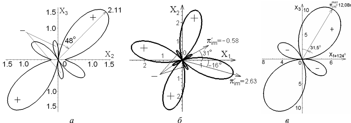
Рис. 5. Перерізи головними площинами ВП поздовжнього ПОЕ \pi'_{ii} кристалів ніобату літію (а), вольфрамату кальцію (б) та переріз площиною X_3, X_{1+124^\circ} поперечного ПОЕ p'_{im}^{(m)} кристалів ТГС (в); усе в од. Бр
