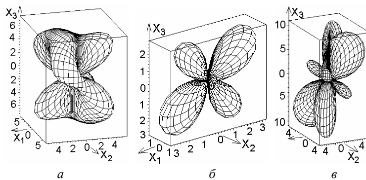
Рис. 4. Вказівні поверхні поздовжнього \pi'_{ii} (а) і поперечного \pi'^{(i)}_{im} (б), \pi'^{(m)}_{im} (в) ПОЕ в моноклінних кристалах тригліцинсульфату ТГС (клас симетрії 2 ); усе в од. Бр
