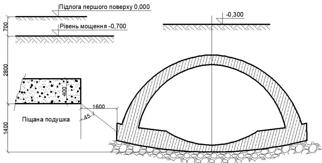
Рис. 3. Профіль нового зміщеного склепіння (розташування нового русла річки Полтви відносно фундаментів)
