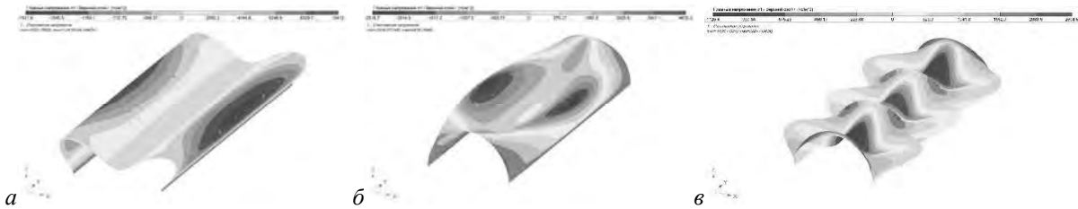
Рис. 9. Ізопля головних напружень \sigma_1 : а – довга оболонка без діафрагм; б – довга оболонка з торцевими діафрагмами; в – довга оболонка з торцевими діафрагмами і проміжними діафрагмами
