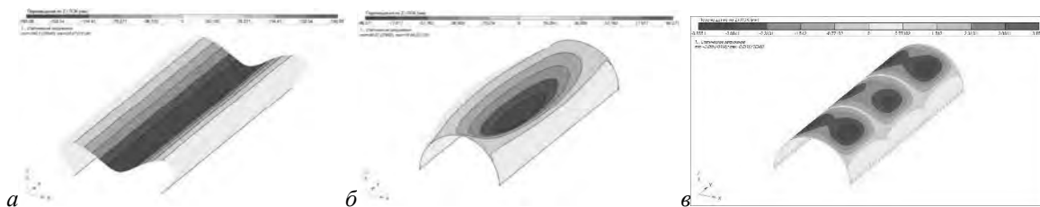
Рис. 11. Ізопля вертикальних переміщень: а – довга оболонка без діафрагм; б – довга оболонка з торцевими діафрагмами; в – довга оболонка з торцевими діафрагмами і проміжними діафрагмами
