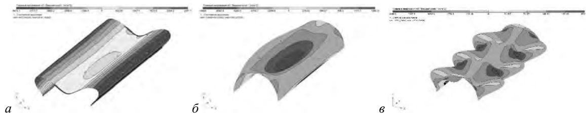
Рис. 10. Ізопля головних напружень \sigma_3 : а – довга оболонка без діафрагм; б – довга оболонка з торцевими діафрагмами; в – довга оболонка з торцевими діафрагмами і проміжними діафрагмами
