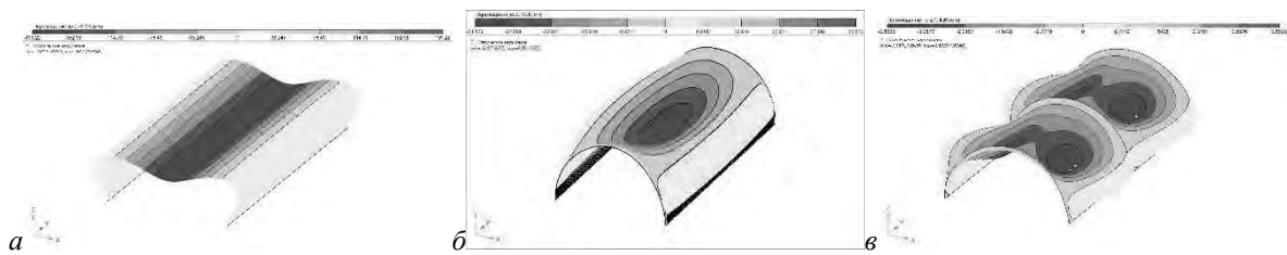
Рис. 8. Ізопля вертикальних переміщень: а – оболонка середн. довжини без діафрагм; б – оболонка середн. довжини з торцевими діафрагмами; в – оболонка середн. довжини з торцевими діафрагмами і проміжними діафрагмами
