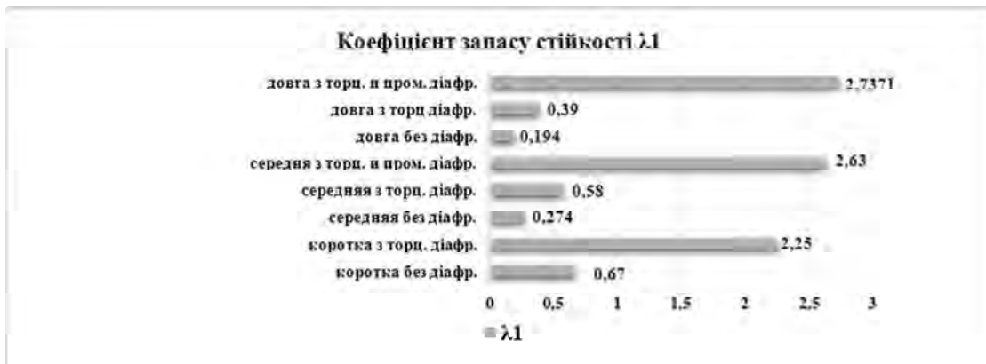
Рис. 12. Порівняльна діаграма коефіцієнтів запасу стійкості \lambda_1
