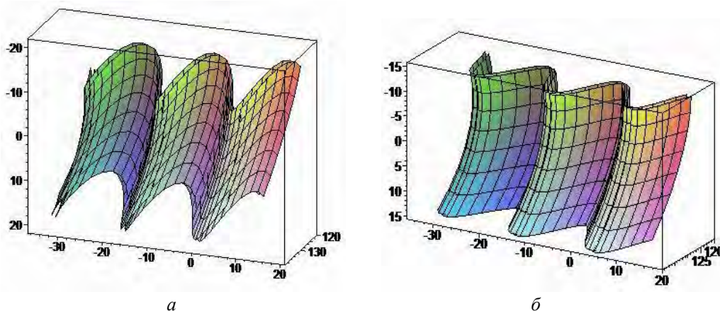
Рис. 3. Бокова поверхня зубців ГК, отримана ДФ способом КРД (а) та ЗПРД (б) (m=5,16 мм; Z_2 = 50 ; R_1 = 31 мм; e = 6,0 мм; r = 6,0 мм; v = 105^\circ ; B = 1 мм; R_{p2} = 122,55 мм, R_{r2} = 129,00 мм, R_{m2} = 128,55 мм, A_m = 158,55 мм)
