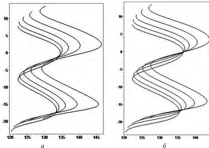
Рис. 5. Січні профілі поверхонь зубів ГК, утворені ДФ способом ЗПРД ( R_1 = 30 мм; r = 6,0 мм; B = 0 мм; R_{m2} = 128,55 мм; A_m = 158,55 мм; m = 5,16 мм; Z_2 = 50 ) (а) ( R_1 = 40 мм; r = 7,0 мм; B = 0 мм; R_{m2} = 129,55 мм; A_m = 169,55 мм; m = 5,16 мм; Z_2 = 50 ) (б)
