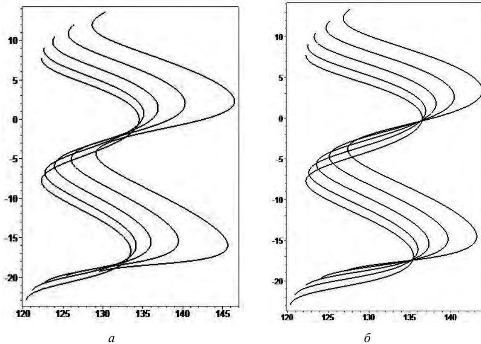
Рис. 4. Січні профілі поверхонь зубів ГК, утворені ДФ способом КРД ( R_1 = 30 мм; e = 6,0 мм; B = 0 мм; R_{m2} = 128,55 мм; A_m = 158,55 мм; m = 5,16 мм; Z_2 = 50 ) (а) ( R_1 = 40 мм; e = 7,0 мм; B = 0 мм; R_{m2} = 129,55 мм; A_m = 169,55 мм; m = 5,16 мм; Z_2 = 50 ) (б)
