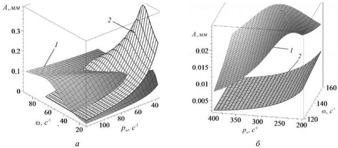
Рис. 5. Залежність величин складових амплітуди коливань муфти A_{\nu q} - 1, A_{\nu g} - 2 від її власної частоти та частоти збудника, h_x = 0,1, h_m = 0,3 : а – “м’яка” муфта, випадок p_x = \Phi ; б – “жорстка” муфта
