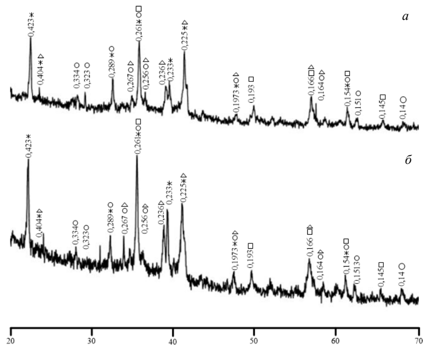
Рис. 3. Дифрактограми цементного каменю із додатком 2 % активованого вапна після 7 (а) та 28 (б) діб тверднення, * - C_2S , o - C_3S , □ - портландит, Δ - еtringіт
