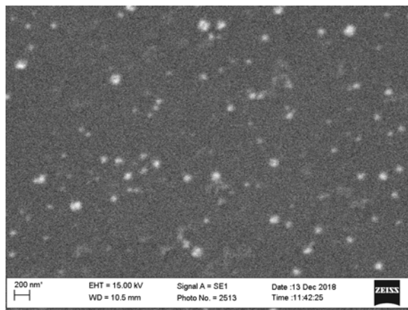
Рис. 2. SEM зображення поверхні кремнію з наночастинками золота, осадженими гальванічним заміщенням із розчинів 2 мМ \text{HAuCl}_4 в ДМСО
