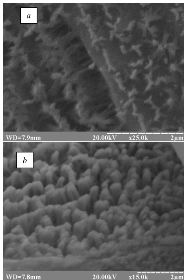
Рис. 4. SEM-зображення нанодротів (a) та нанодротів кремнію (b)
