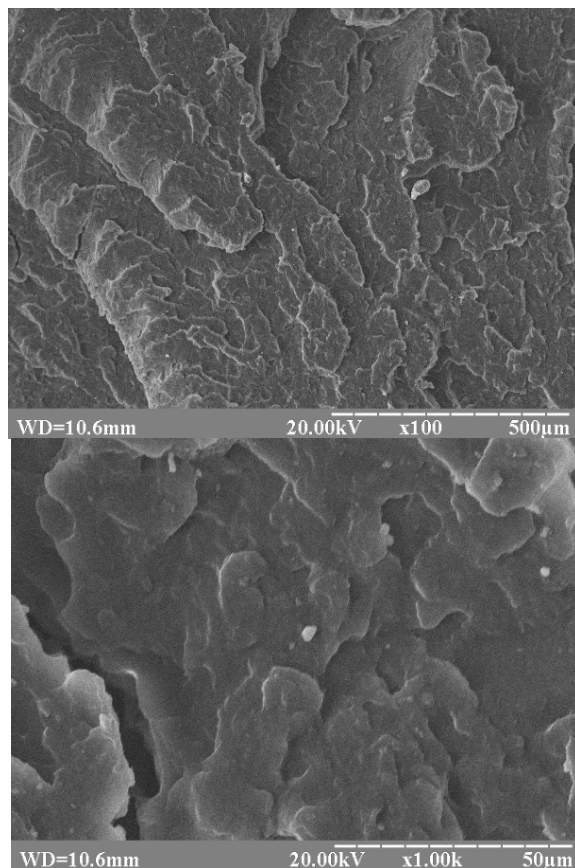
Рис. 3. Мікрофотографія поверхні вихідного поліпропілену
