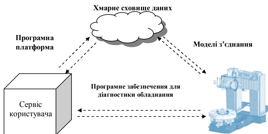
Основні програмні елементи системи
