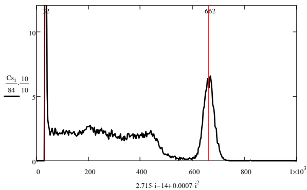
Рис. 2. Апаратурний відгук спектра від точкового джерела ^{137}\text{Cs} для гамма-детектора CsI
