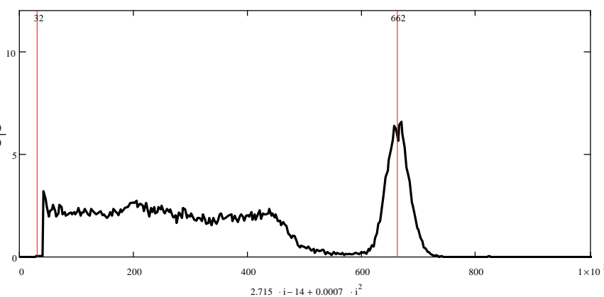
Рис. 5. Апаратурний відгук спектра для гамма-детектора CsI від ДІВ ^{137}\text{Cs} у тонкій капсулі зі сталі на установці УПД-2
