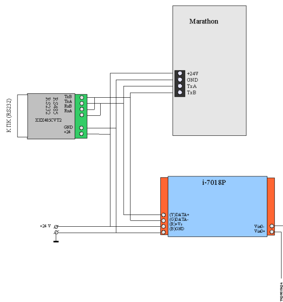
Рис. 3. Структурна схема інтерфейсного блока для експериментальних вимірювань
