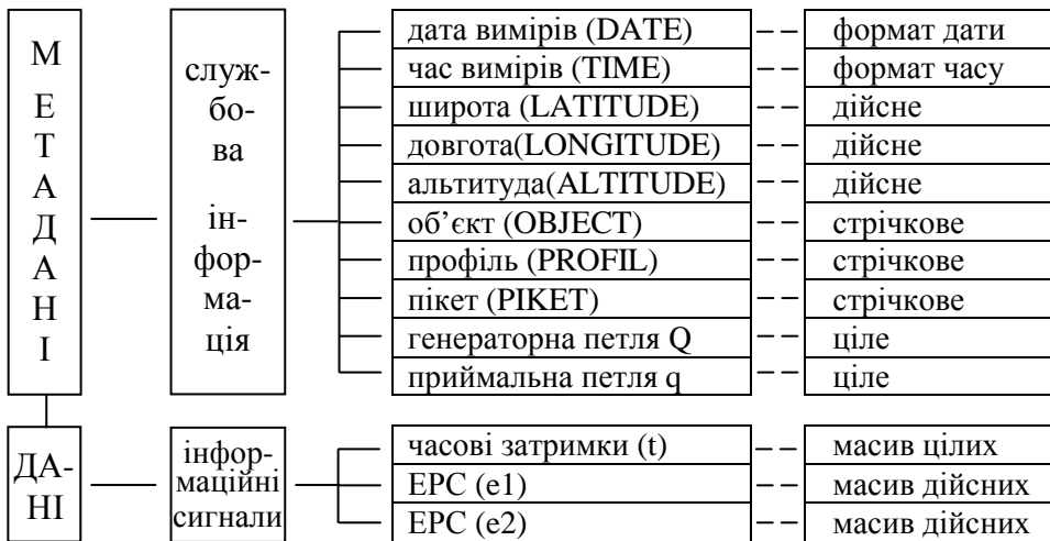
Рисунок 7 – Інформаційна модель структуризації даних ЗСБ
