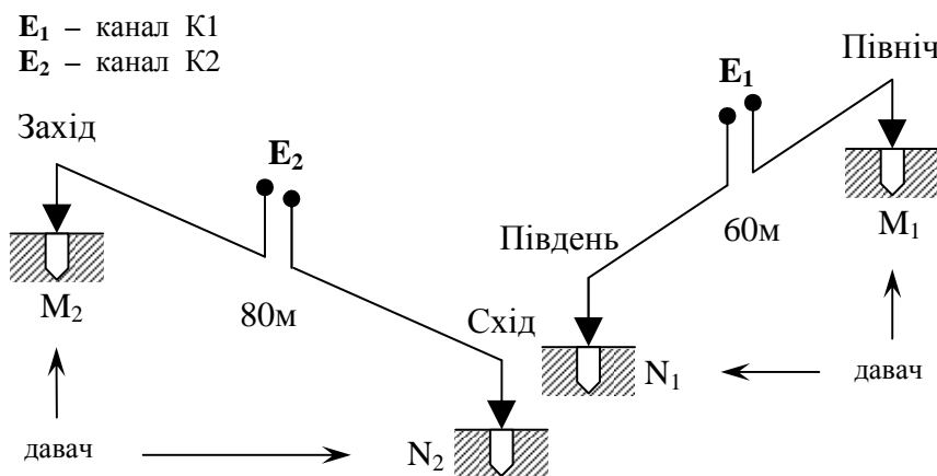
Рисунок 1 – Схема вимірювальної установки
