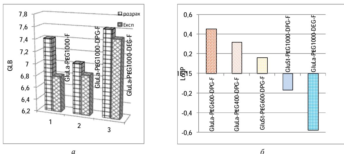
Рис. 3. Залежність коефіцієнта розподілу ( \log(P) ) від структури кополіестерів: а – порівняння кополіестерів, синтезованих без низькомолекулярного комономеру (1) та з дипропіленгліколем (2) або диетиленгліколем (3); б – порівняння коефіцієнта розподілу ( \log P ) для кополіестерів різного складу (зразки 3,1,6,9,11, табл. 2)
