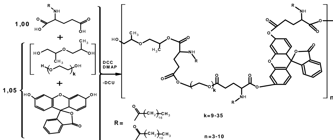
Рис. 1. Схема отримання флуоресцеїнвмісного кополіестеру при кополіконденсації його з N-заміщеною глутаміновою кислотою і політердіолами за реакцією Стегліха
