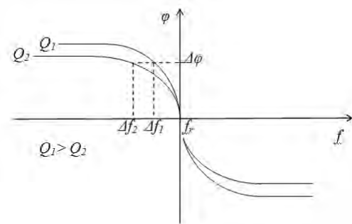
Рис. 2. Фазочастотна характеристика коливального контуру
