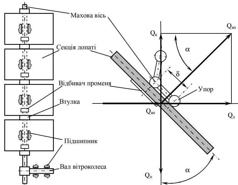
Рис. 1. Вітродвигун (а) та схема самоналаштування секції лопаті (б): Q_{вп} – сила вітрового потоку; Q_к – сила обертання; Q_п – сила опору зустрічного потоку повітря; Q_д – сила тиску на секцію лопаті; \alpha – кут самоналаштування секції лопаті; d – ексцентриситет
