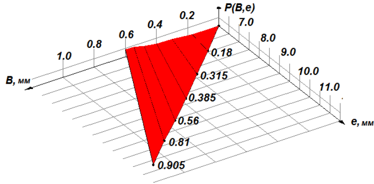
Рис. 5. Полігон щільності розподілення мішаного масиву значень складального зазору “B” та ширини шва “e”
