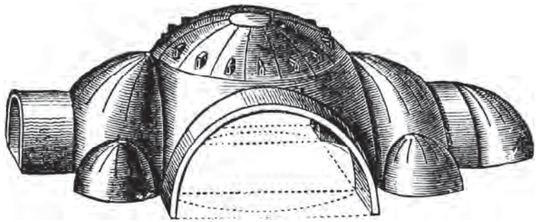
Рис. 15. Собор св. Софії у Константинополі. Схема конструктивної системи перекрить
