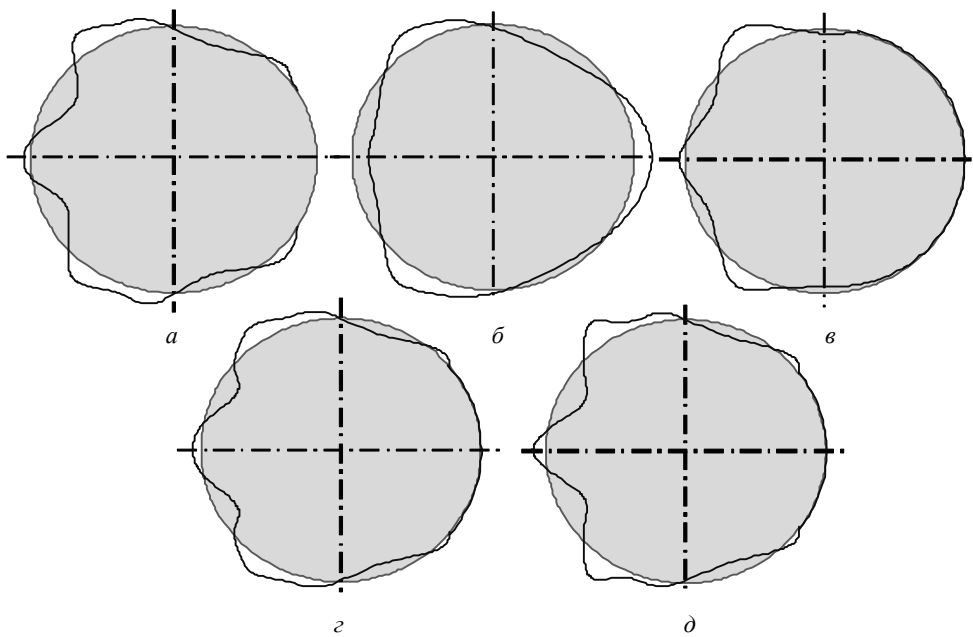
Рис. 8. Характер деформування ємностей, підкріплених вертикальними ребрами жорсткості, за дії асиметричного навантаження за епюрою вітрового тиску при D_w=1 :
