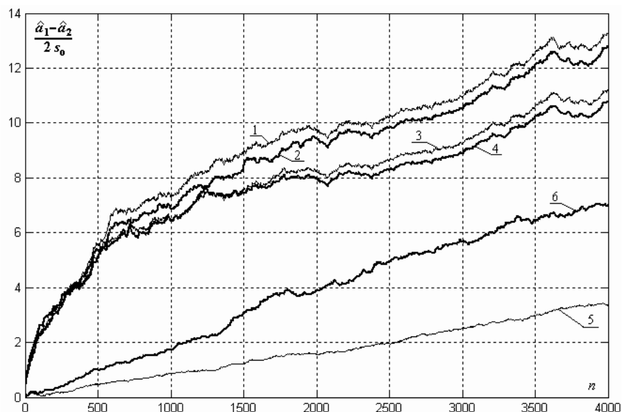
Рис. 2. Залежність ефективності оброблення від розміру вибірки n для: 1 – диференційної ентропії обчисленої за дисперсією без інтерполяції; 2 – диференційної ентропії обчисленої за дисперсією з інтерполяцією; 3 – СКВ без інтерполяції; 4 – СКВ з інтерполяцією; 5 – ентропії за Шенноном без інтерполяції; 6 – ентропії за Шенноном з двократною інтерполяцією
