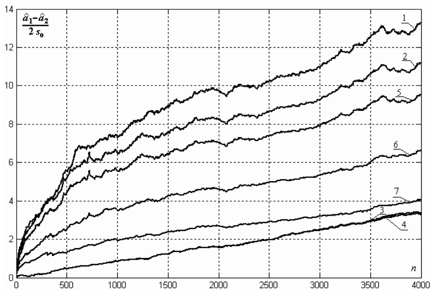
Рис. 1. Залежність ефективності оброблення від розміру вибірки n для:
