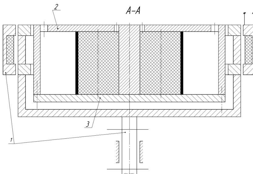
Fig. 3. Section A-A
