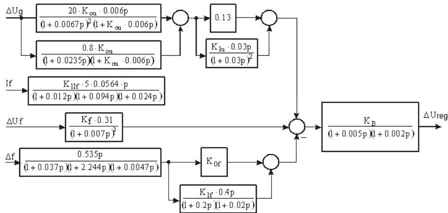
Рис. 2. Структурна схема регулятора збудження типу APB-СД
