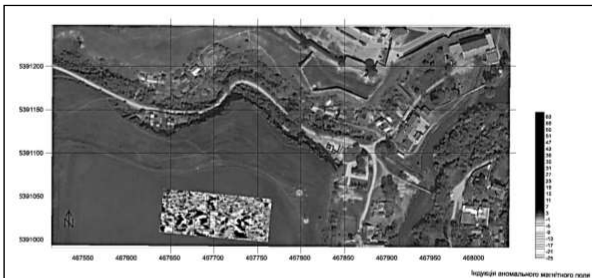
Рис. 2. Карта індукції магнітного поля та її географічне положення в межах ділянки «Хрест» (за О. А. Лошаковим)
