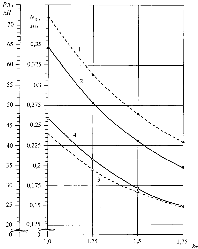
Рис. 4. Вплив коефіцієнта запасу міцності тіла шарошки на величину оптимального натягу пресового з’єднання „зубок–шарошка” та на силу випресовування зубка на різних ділянках хвостовика: 1 – сила випресовування у ділянці спряження „твердий сплав – сталь”; 2 – величина натягу в ділянці спряження „твердий сплав – сталь”; 3 – сила випресовування у ділянці спряження „сталь – сталь”; 4 – величина натягу в ділянці спряження „сталь – сталь”
