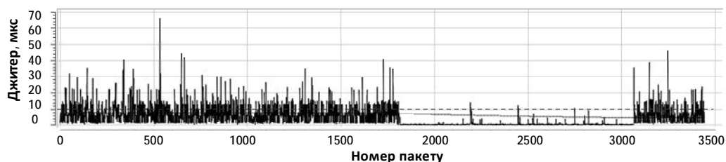
Рис. 5. Джитер IPTV потоку в маршрутизаторі
