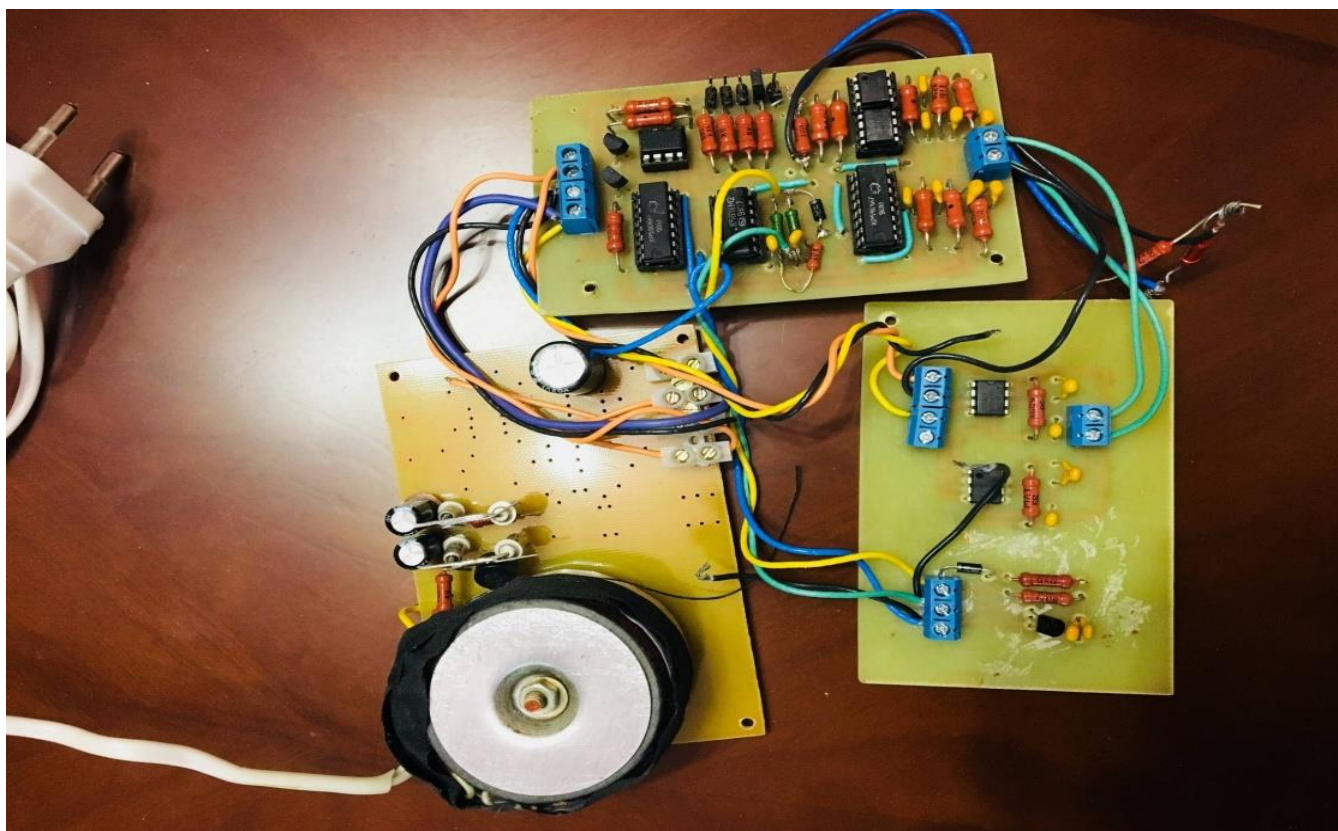
Рисунок 4.9 – Зовнішній вигляд макету калібратора напруги з додатковим джерелом зразкової напруги та аналоговою пам'яттю
