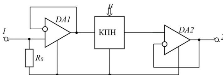
Рисунок 1.11 – АІО з функцією перетворення R_{ім} = R_0(1 - \mu)
