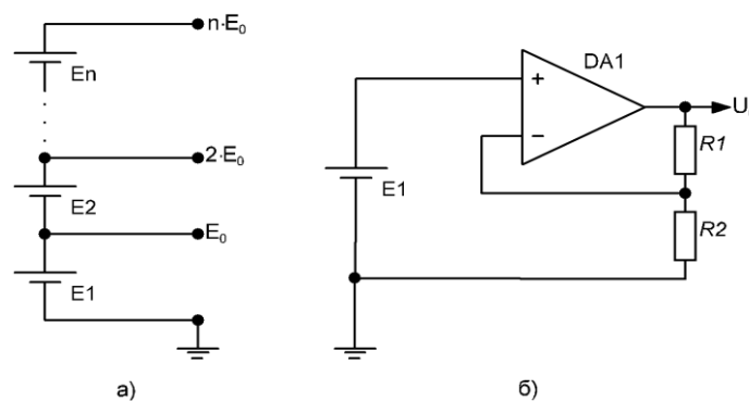
Рисунок 1.5 – Багатозначна міра напруги на: а) послідовно з'єднаних однозначних зразкових мірах; б) з додатковим підсиленням
