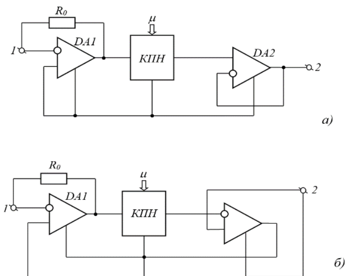
Рисунок 1.12 – АІО з функцією перетворення R_{ім} = R_0 \mu
