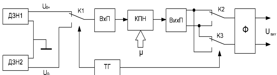
Рисунок 2.5 – Структурна схема калібратора напруги з додатковим джерелом зразкової напруги
