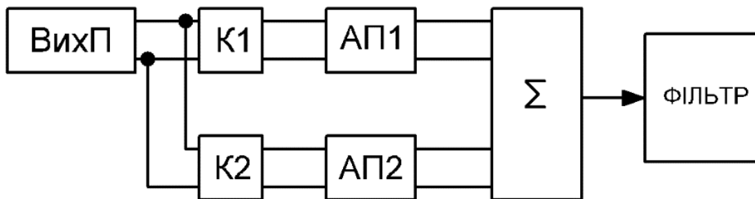
Рисунок 2.10 – Структурна схема вихідної частини калібровача напруги постійного струму з елементами аналогової пам'яті
