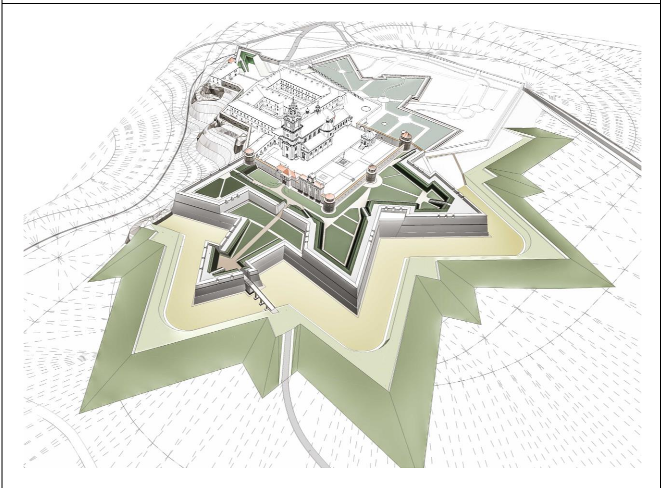
Рис. 4. Пропозиція комплексної реставрації оборонних споруд монастиря оо. Домініканів у Підкамені
