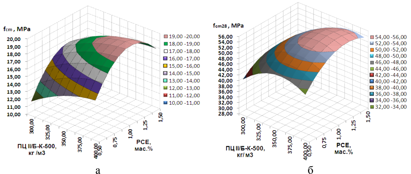
Рисунок 4 - Ізопараметричні діаграми зміни міцності на стиск модифікованих бетонів через 2 (а) та 28 (б) діб тверднення
