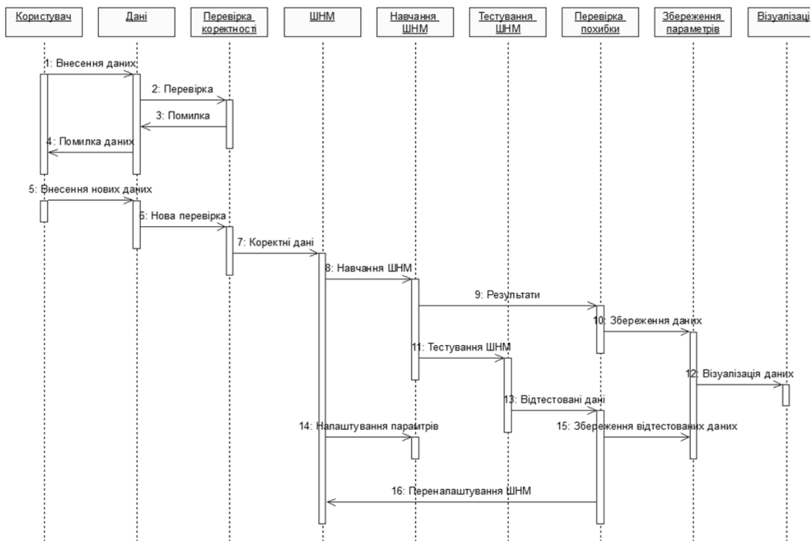
Рис 2. Діаграма послідовності
