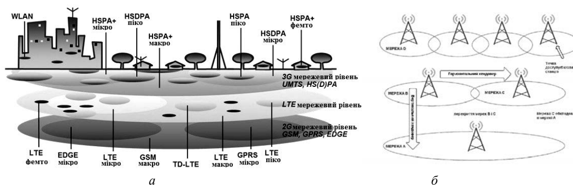
Рис. 1. Архітектура гетерогенної мережі (HetNet)(а) та вертикальний і горизонтальний хендовер (б)
