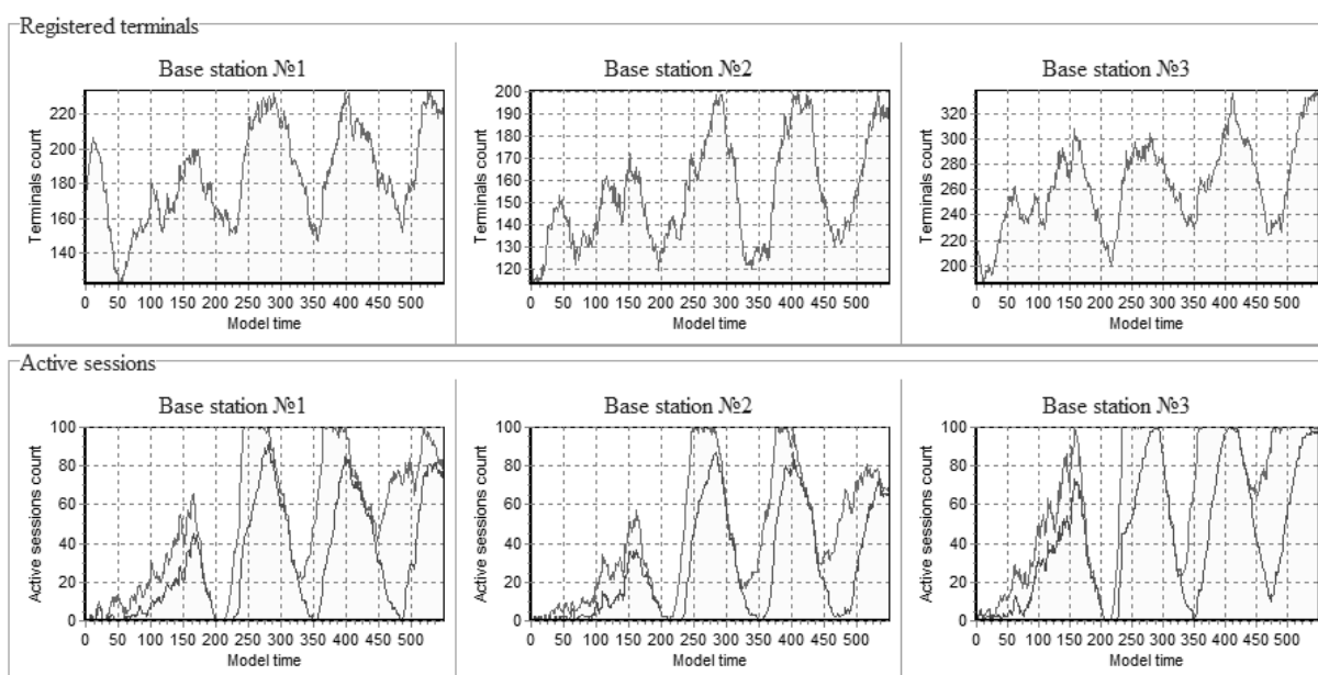
Рис. 8. Часові характеристики роботи UMTS в умовах перевантаження системи GSM у гетерогенній мережі
