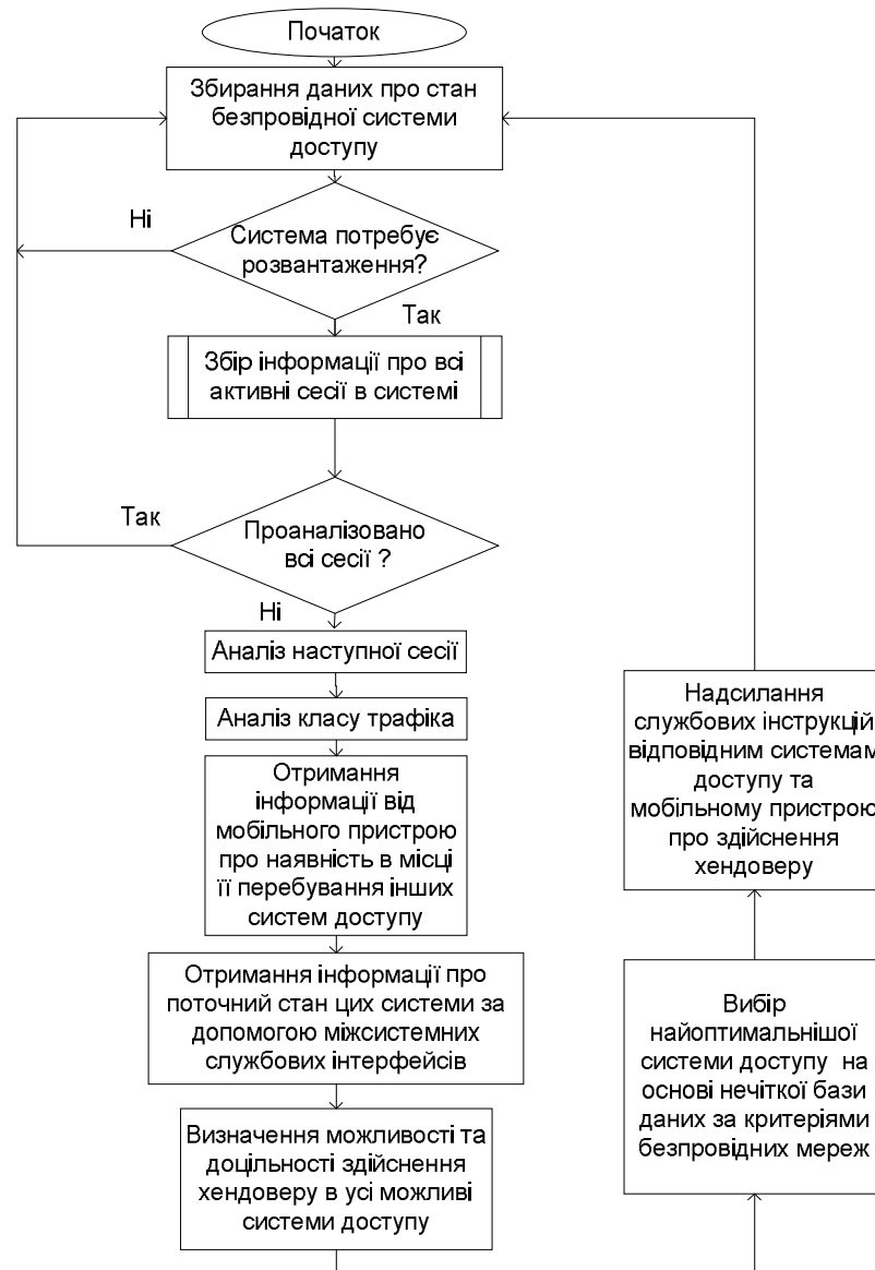
Рис. 3. Алгоритм роботи централізованого інтелектуального вертикального хендверу
