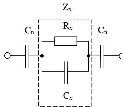
Рис. 1. Схема заміщення системи “сенсор–вимірювальний засіб”: Z_x – імпеданс об'єкта контролю (овочевого соку); C_n – приелектродний імпеданс
