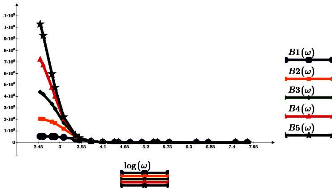
Рис. 7. Графік залежності реактивної складової B(\omega) від частоти тестового сигналу (Гц) за різних значень опору об'єкта контролю. C_n = 18 \text{ мкФ} , C_x = 1500 \text{ нФ} , R_x = 20, 40, 60, 80, 100 \text{ Ом}
